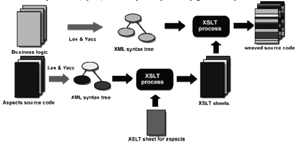
Figura 1. Proceso de Tejido de phpAspect
